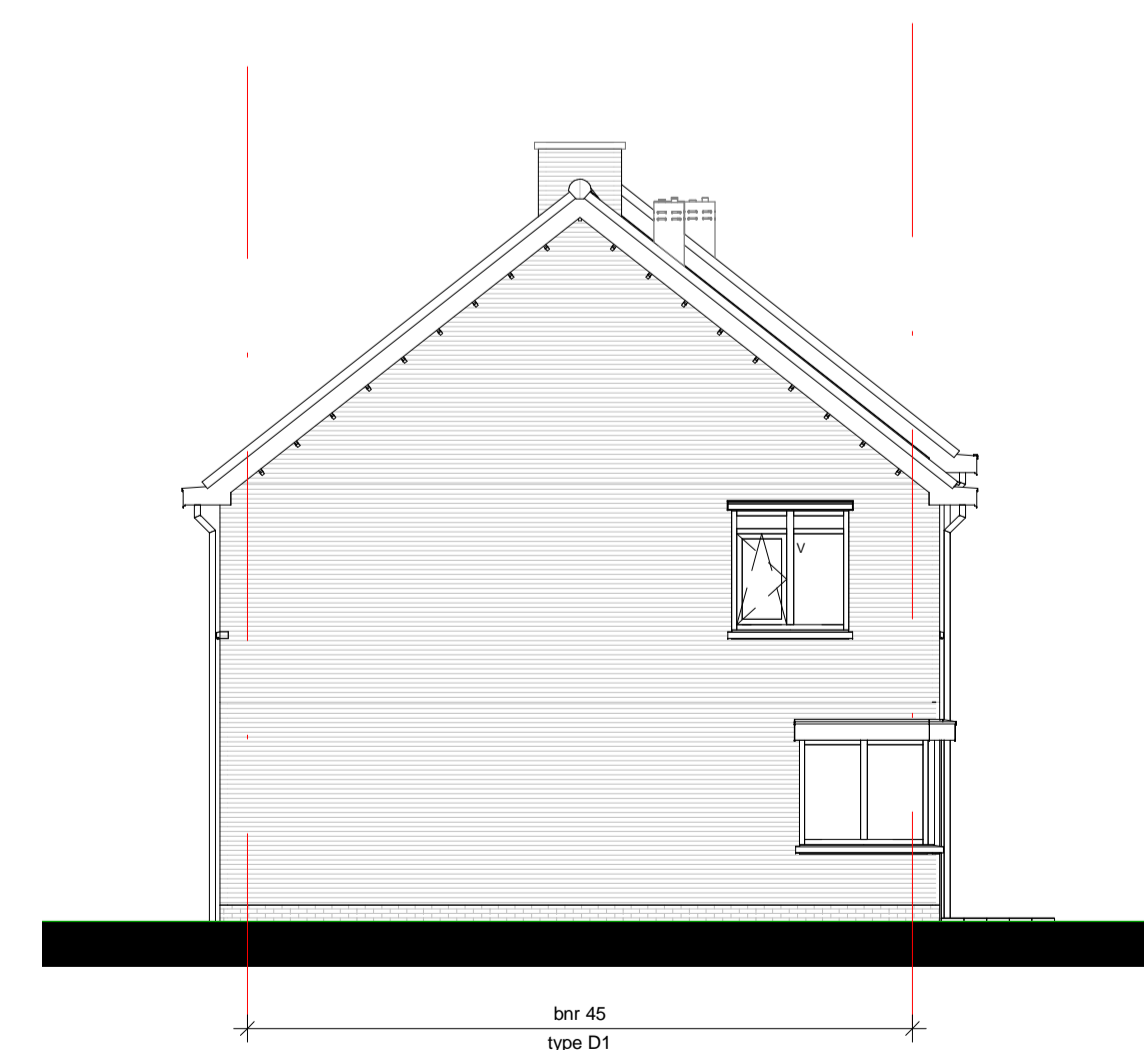
Linkerzijgevel
