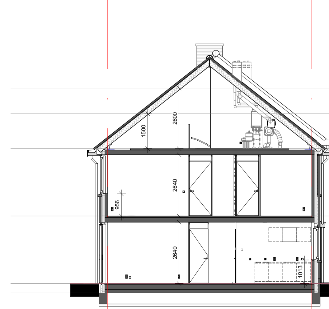
Doorsnede A
