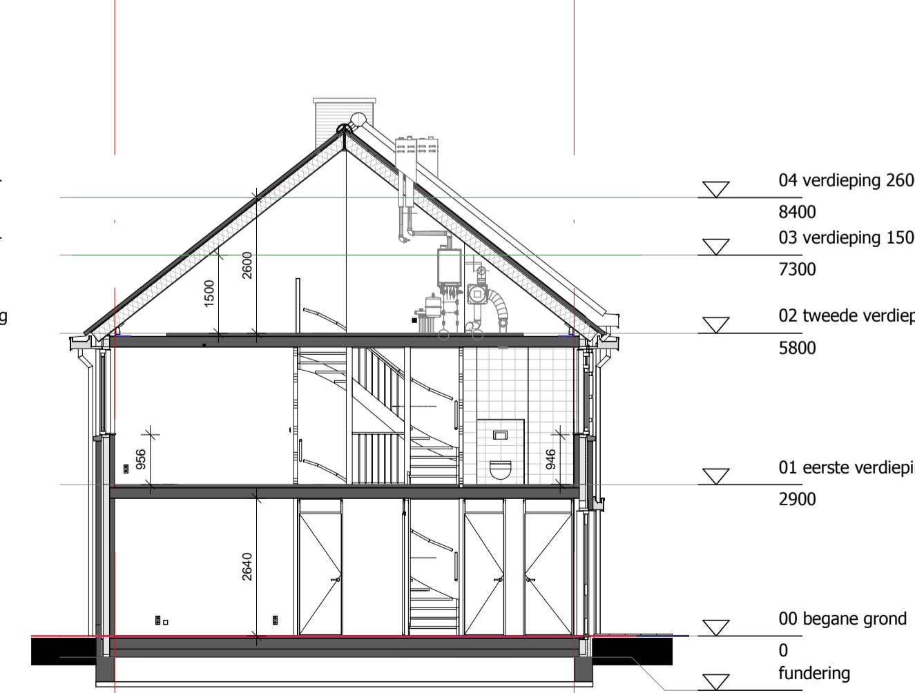
Doorsnede B
