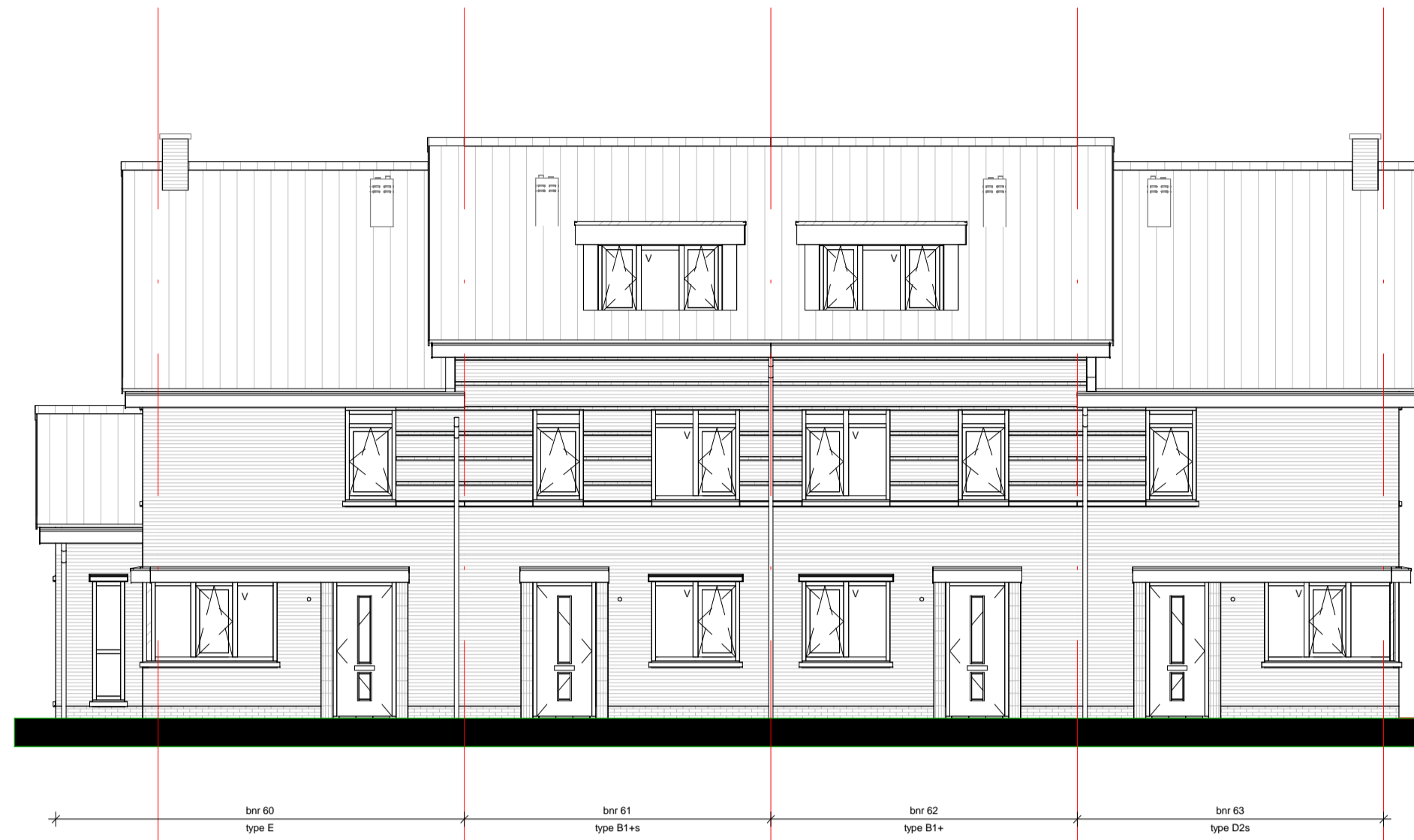
Voorgevel schaal 1 : 100
