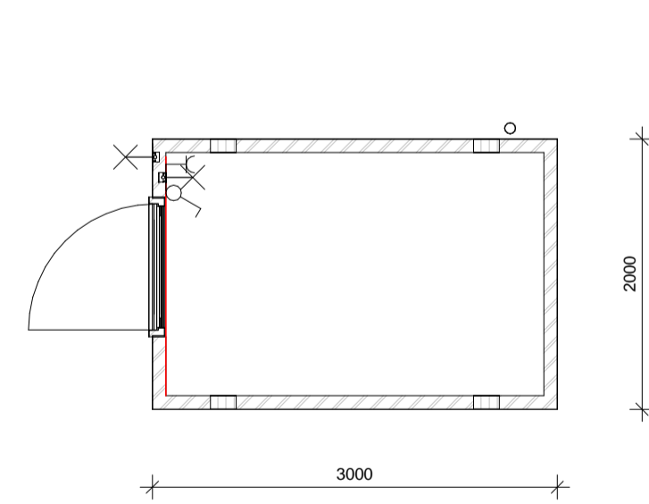
Metselwerk berging
