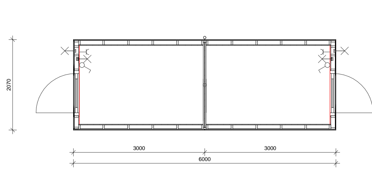
Dubbele berging hout
