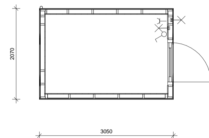
Metselwerk berging
